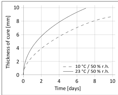
圖表 1: Sikaflex®-227 固化速率
