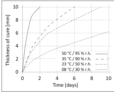
圖表 1: 固化速率 Sikasil® SG-20
