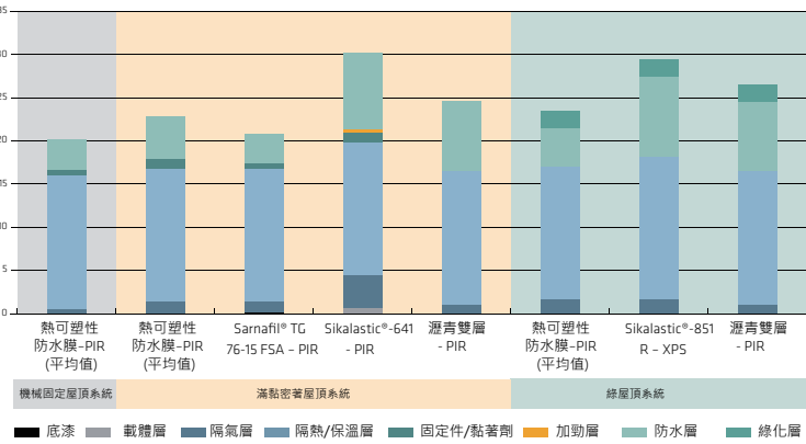
常見的屋頂系統之LCA 結果 1) 每平方公尺屋頂系統之GWP(全球暖化潛能) (kg CO 2 -eq./m 2 )
