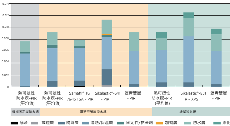
常見的屋頂系統之LCA 結果 1) 每平方公尺屋頂系統之光化學臭氣產生潛能 [kg C 2 H 4 -eq./m 2 ]
