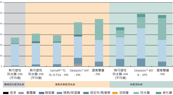
常見的屋頂系統之LCA 結果 1) 每平方公尺屋頂系統之累積能源需求(CED)(MJ/m 2 )
