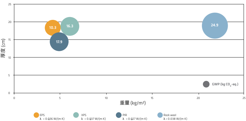
常見的屋頂隔熱解決方案的環保效率 1) 全球暖化潛能(GWP)(kg CO 2 -eq.) 與不同隔熱材料的厚度與重量
